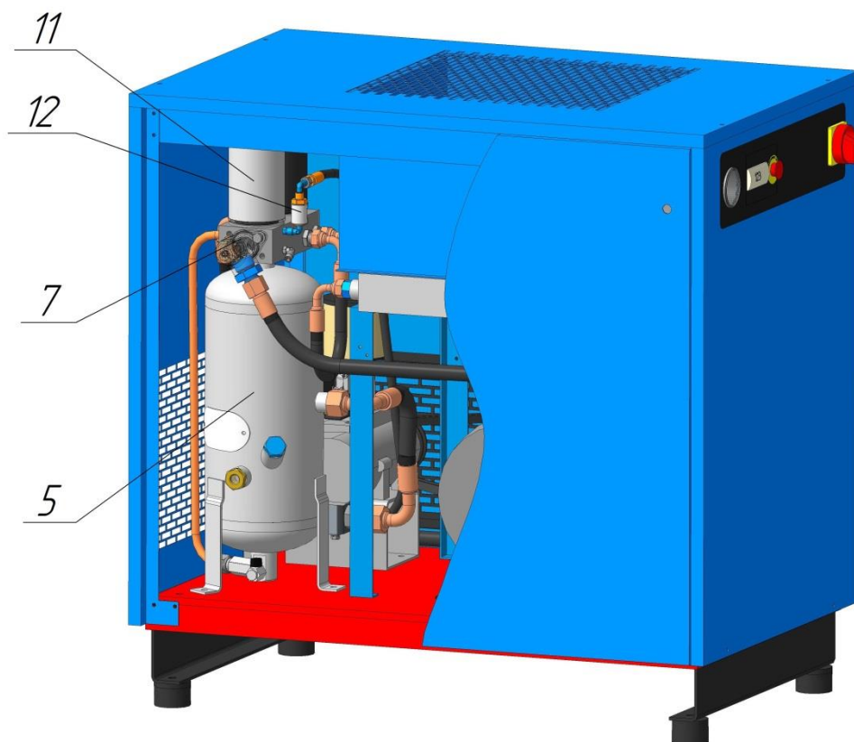
Рисунок 1 – Общий вид компрессорной установки ВК20Т-8(10, 15)
