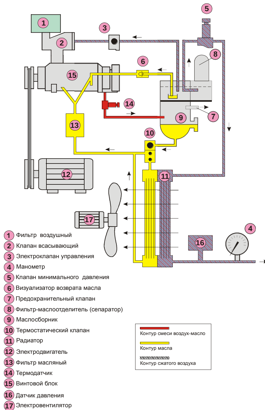
Рисунок5— Схема функциональная принципиальная компрессорной установки
