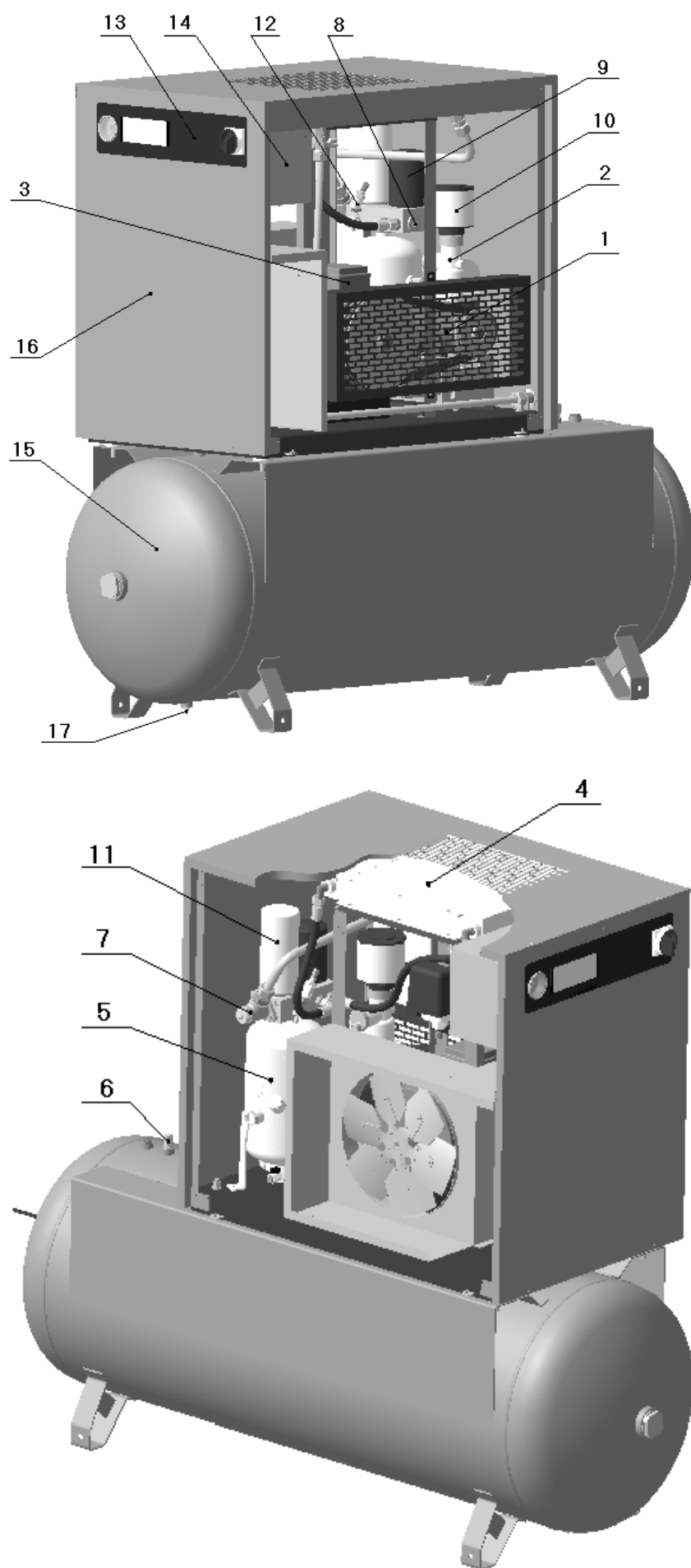
Рисунок 2 – Общий вид компрессорной установки ВК15Т-...-500
