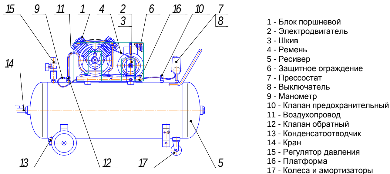
Рисунок 7 - Общий вид компрессора СБ4/С-200.LB30-3.0
