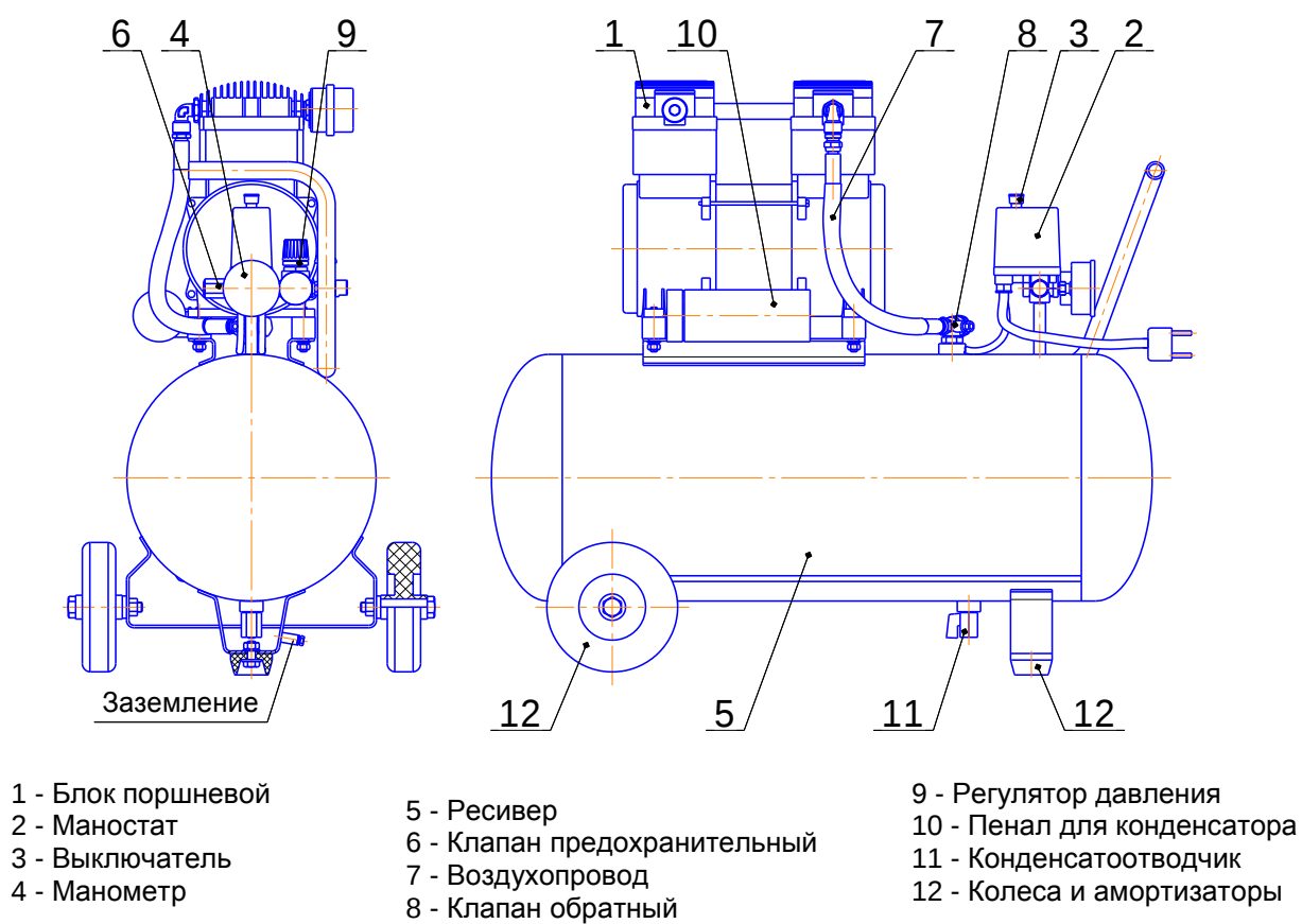
Рисунок 6 - Общий вид компрессоров СБ4/С-50.OLD15, СБ4/С-50.OLD20
