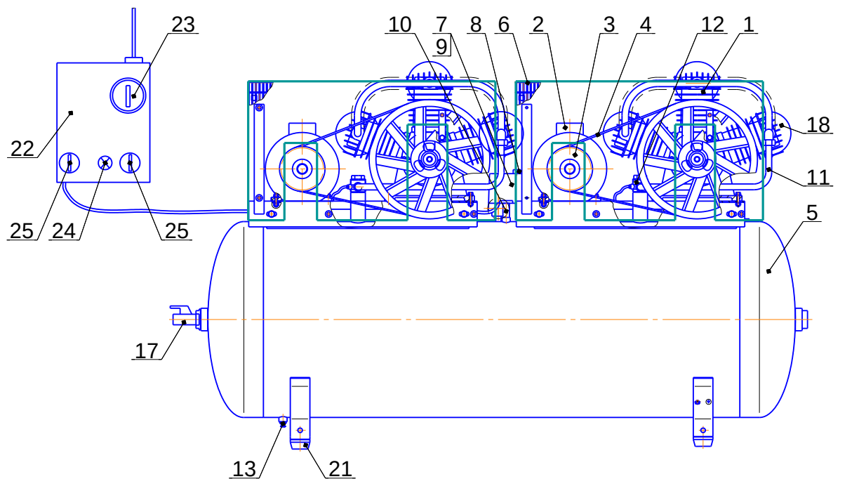
Рисунок 8 - Общий вид компрессора СБ4/Ф-500.LB75ТБ
