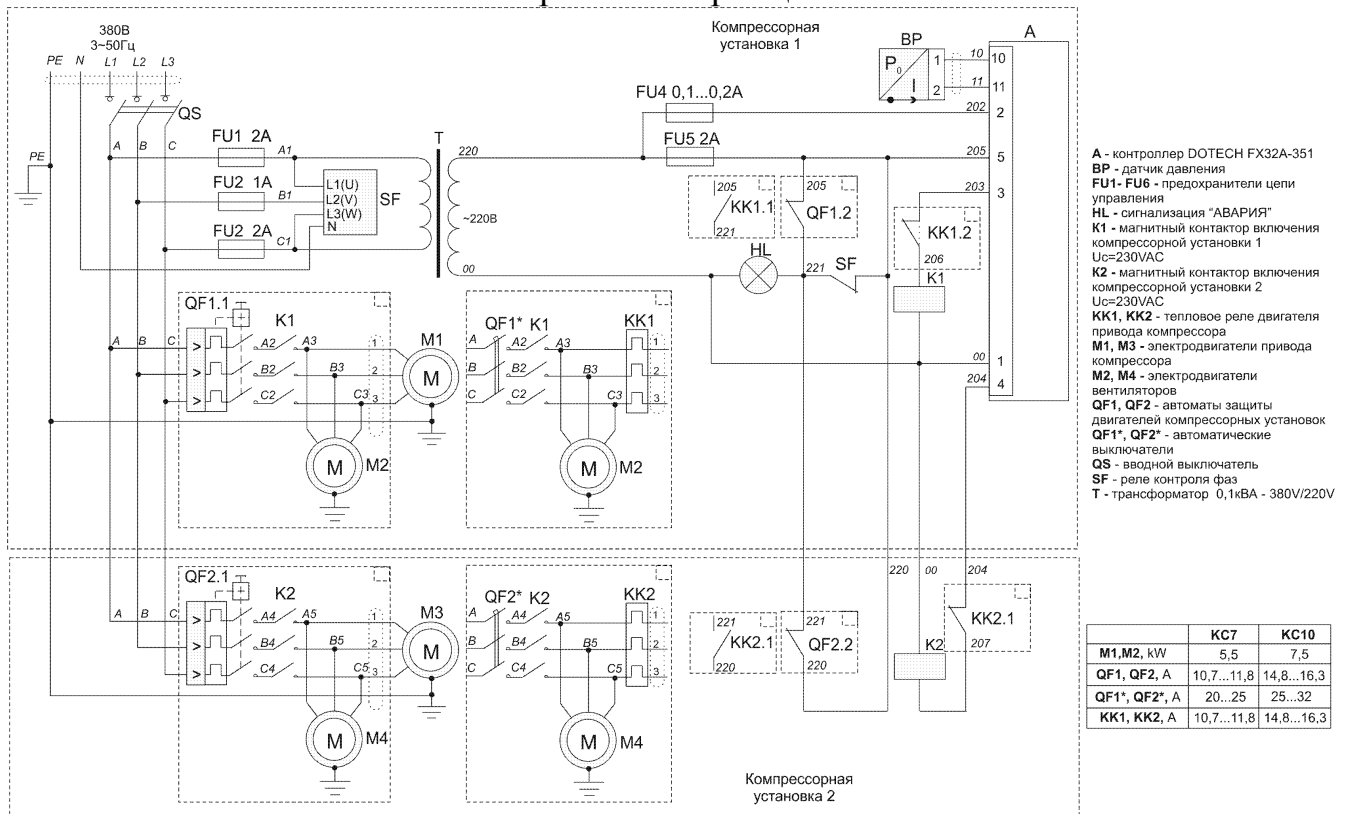
Рисунок Б.1 – Схема электрическая принципиальная компрессорных установок KC7-8-500TM, KC7-8-500-1TM, KC10-8-500TM, KC10-8-500-1TM
