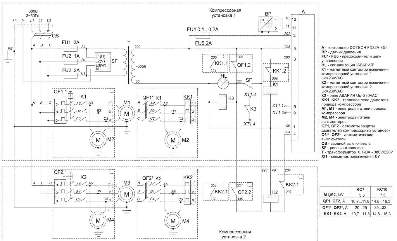
Рисунок Б.2 – Схема электрическая принципиальная компрессорных установок KC7-8-500TM, KC7-8-500-1TM, KC10-8-500TM, KC10-8-500-1TM с дистанционным управлением
