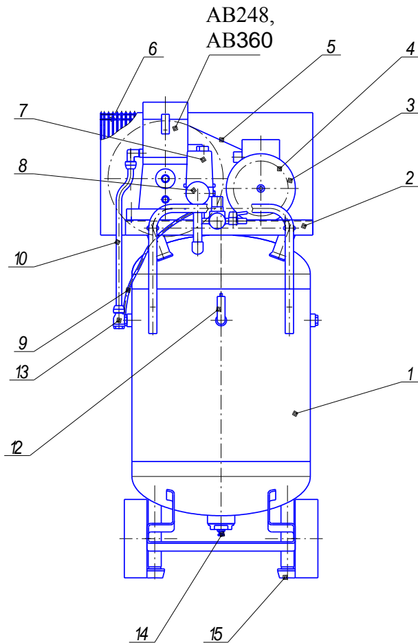
Рисунок 2 – Общий вид компрессора СБ4/С-100.АВ248АВ, СБ4/С-100.АВ360В, СБ4/С-100.АВ360АВ
