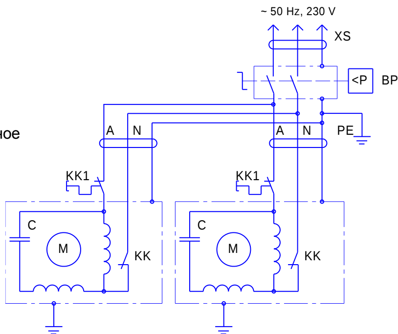
Рисунок А.1 - Схема электрическая принципиальная компрессора СБ4-100.OLD15T
