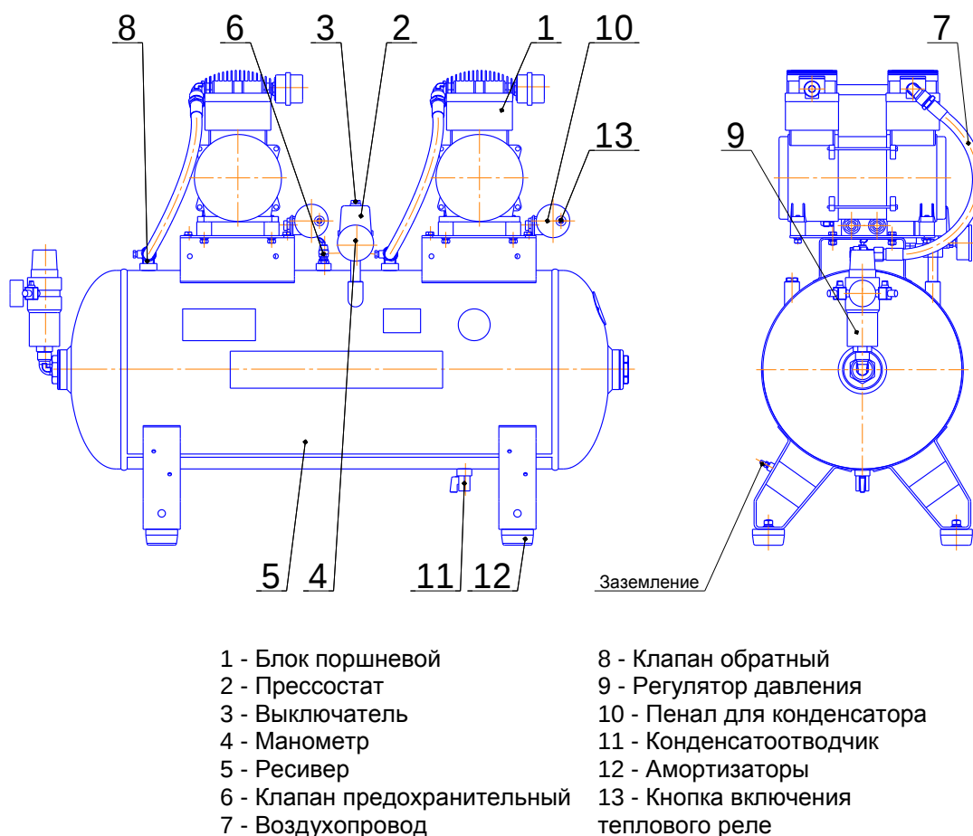
Рисунок 3 - Общий вид компрессора СБ4-100.OLD15T
