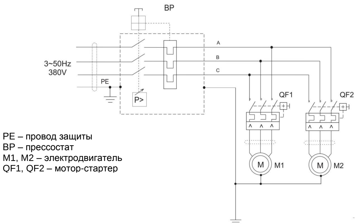
Рисунок А.2 - Схема электрическая принципиальная компрессора СБ4-100.OLD20-3T
