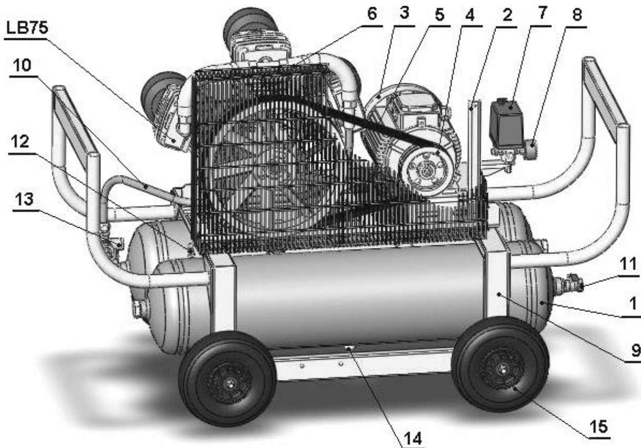
Рисунок 1 – Общий вид компрессора СБ4/С-90.ЛВ75
